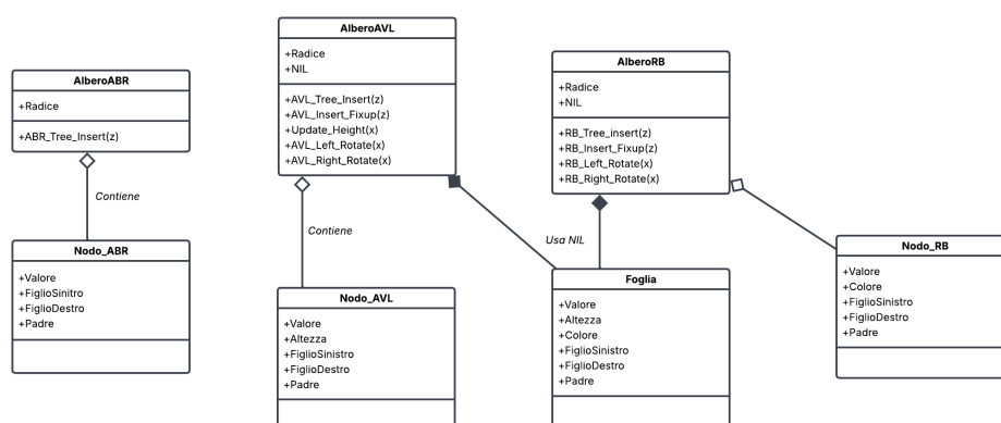
Figura 4: Diagramma delle classi del codice
